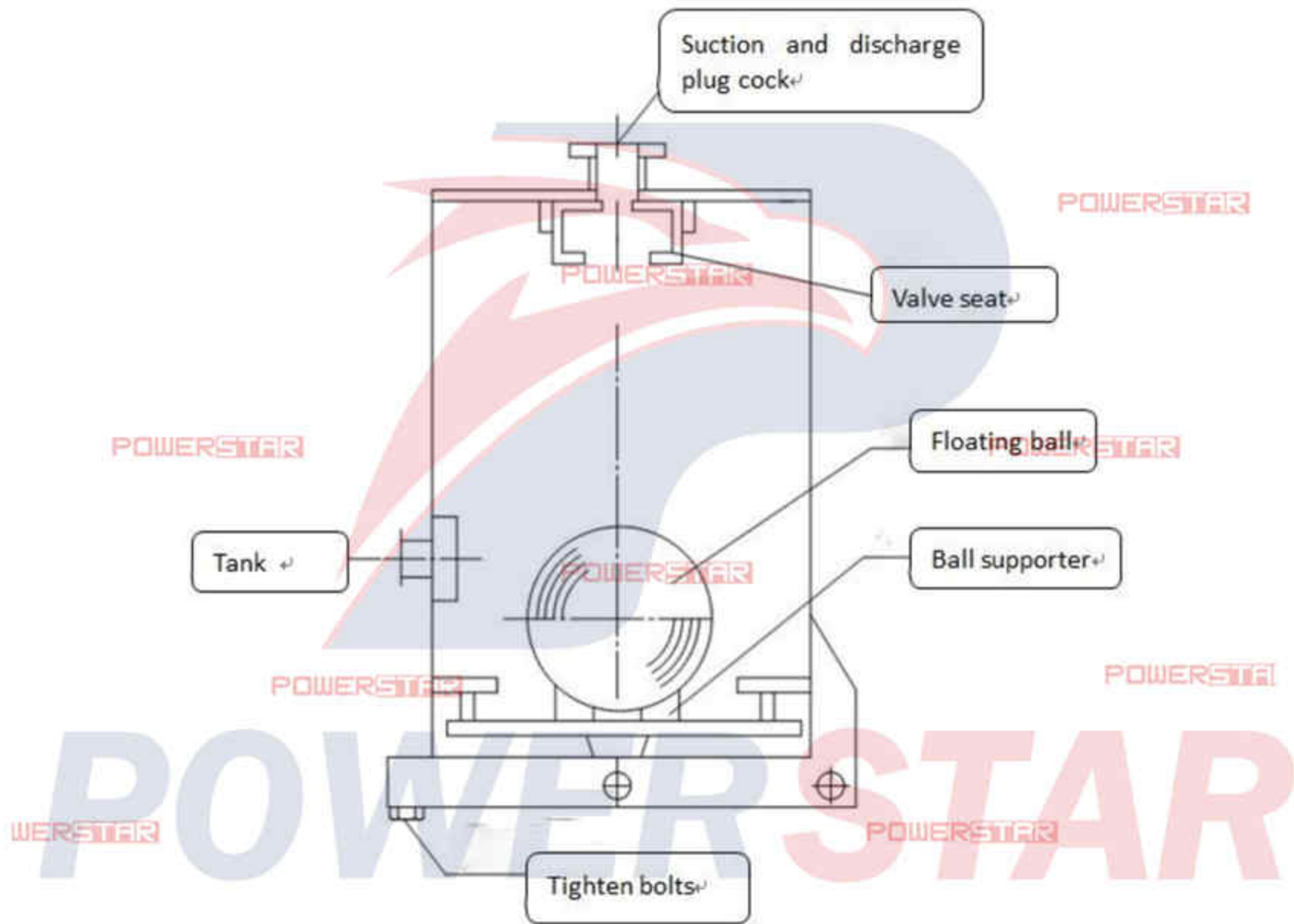
(Water-Gas Separator)
